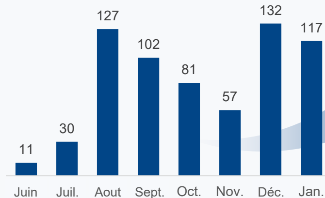
Production mensuelle de clinker du four 6 (kt)
